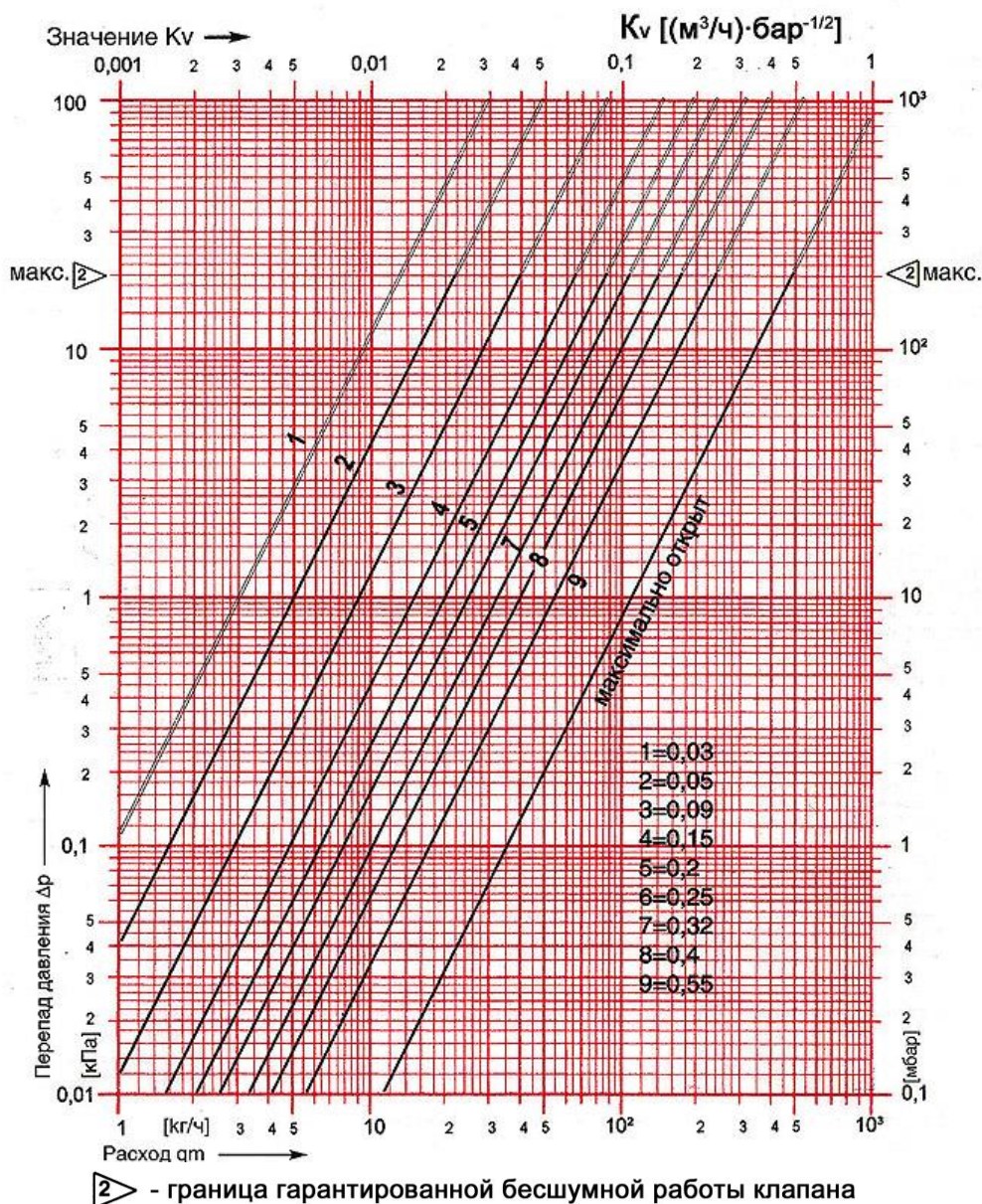
Рис. 2.4. Гидравлические характеристики термостатов «HERZ-TS-90-V» с присоединительными размерами 3/8" и 1/2" с настройкой на режим 2К (2°C) и при снятой термостатической головке (при полном открытии клапана)
