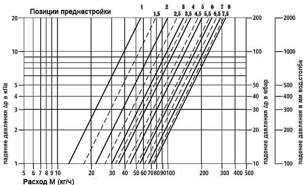
Рис. 2.3. Гидравлические характеристики вентильной вставки V3K S при различных позициях преднастройки при режиме 2K
