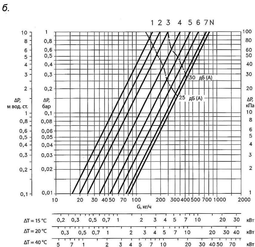
Рис. 2.5. Гидравлические характеристики терморегуляторов «Данфосс» RA-N 15 (а) и RA-N 20/25 (б), предназначенных для двухтрубных систем отопления (при различных уровнях монтажной настройки клапана)
