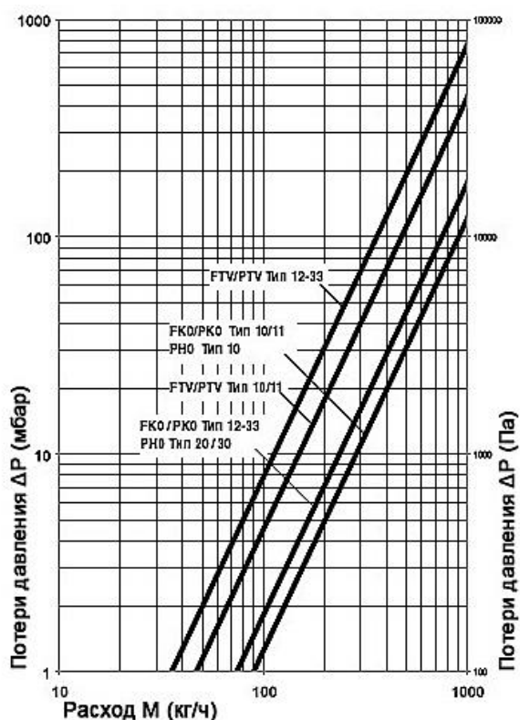
Рис. 2.1. Потери давления в радиаторах «Kermi Therm X2» типов FK0, PK0, FTV, PTV и PNO
