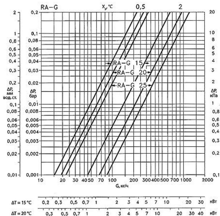
Рис. 2.6. Гидравлические характеристики терморегуляторов пониженного сопротивления «Дanfoss» RA-G при настройке на режимы 0,5К (слева) и 2К (справа)
