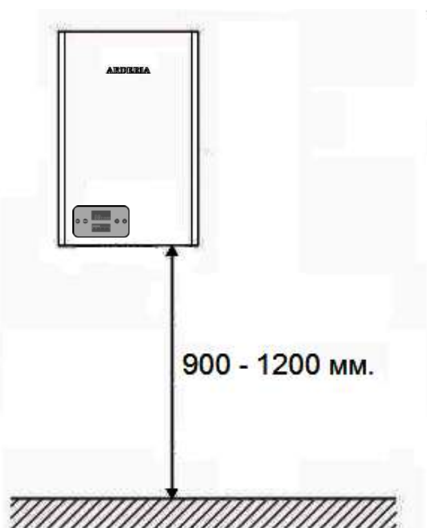
Рис. 10 Монтажные расстояния
