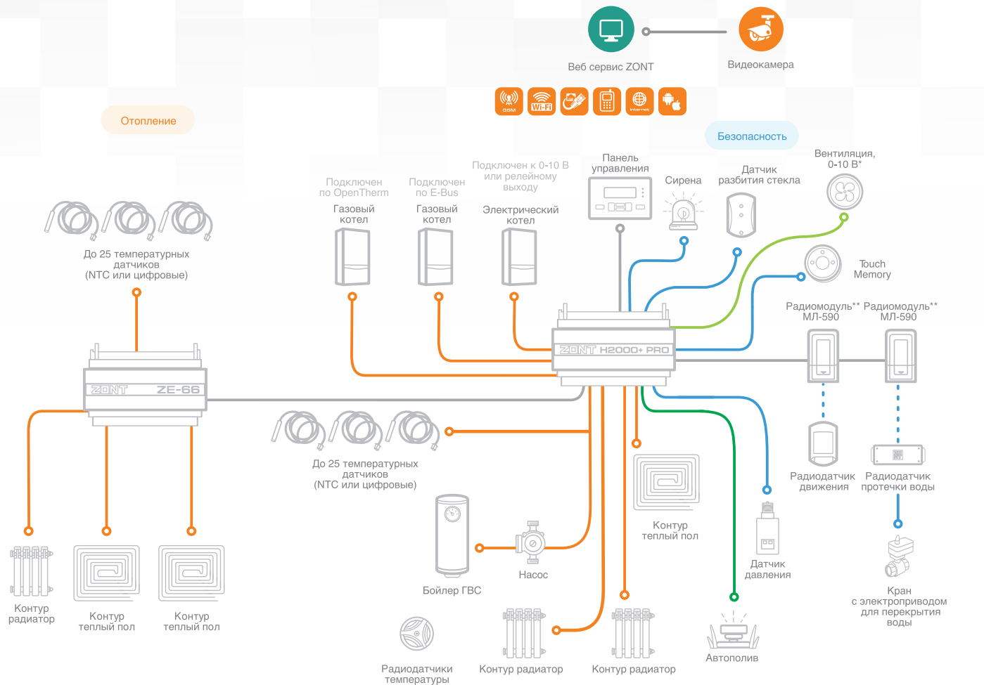
Пример инженерной системы на базе ZONT H2000+ PRO
