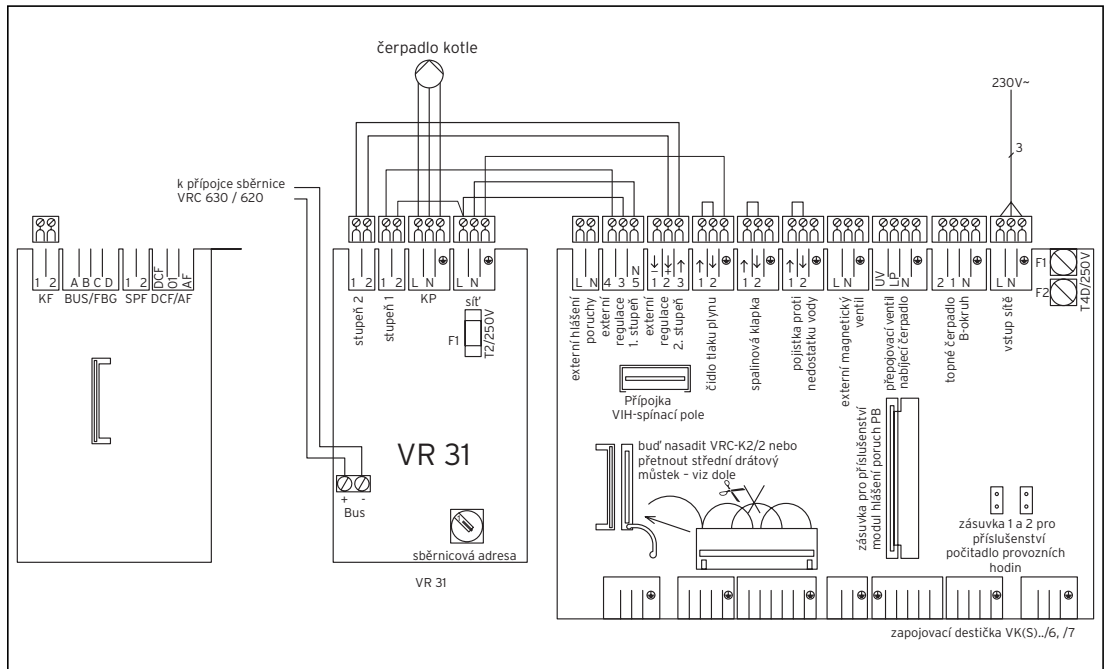
Obr. 4.2 Montážní schéma
