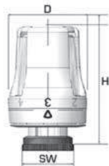
Рис. 6. Габаритные и присоединительные размеры термоголовки Арт. SHT-0002-003015
