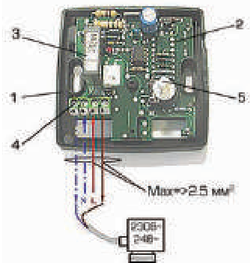
Рис. 8. Устройство электронного термостата
