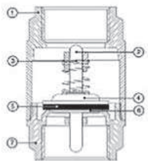
Рис. 30 Устройство обратного клапана с металлическим затвором
