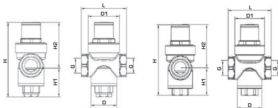
Рис. 21. Редуктор SVS-1009 (1010)
