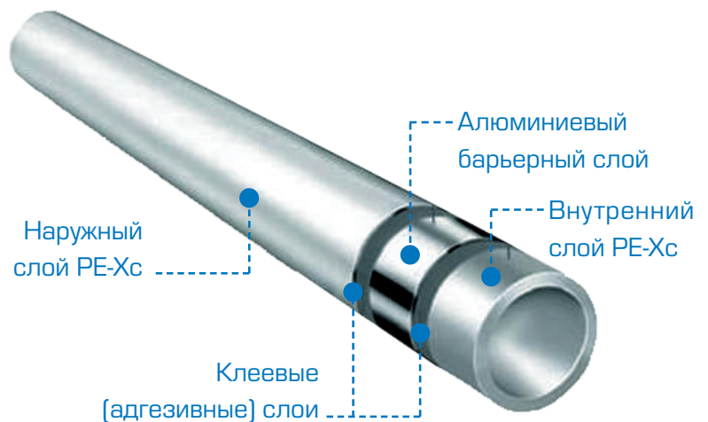
Рис. 2. Пятислойная труба РЕ-Хс/АІ/РЕ-Хс
