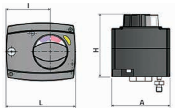
Рис. 6. Габаритные размеры
