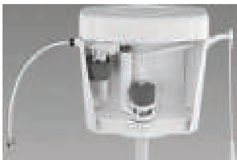
ПОДКЛЮЧЕНИЕ СМЫВНОГО БАЧКА УНИТАЗА
