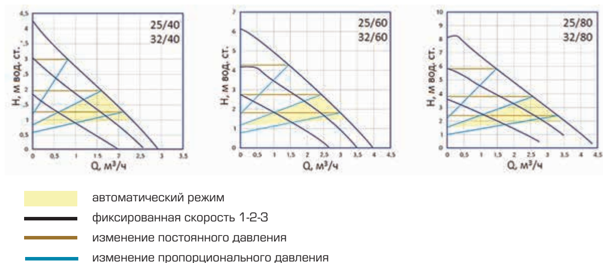
Рис. 11 Расходно-напорные характеристики
