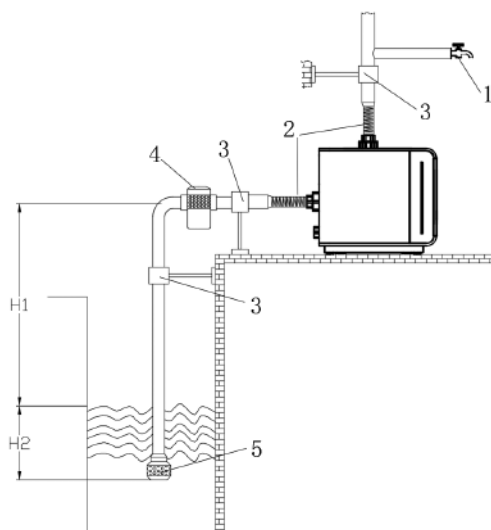
Рис. 5 Схема системы подачи воды из колодца/скважины
