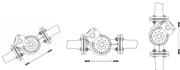
Рис. 28 Возможные положения клеммной коробки
