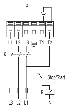
Рис. 31 Схема подключения трехфазного насоса при использовании внешнего механического пускателя ВКЛ/ВЫКЛ
