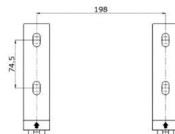
Рис. 9 Монтажные габариты комплекта настенного монтажа
