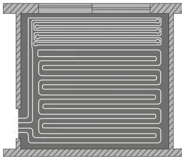
Укладка петель двойной змейкой
