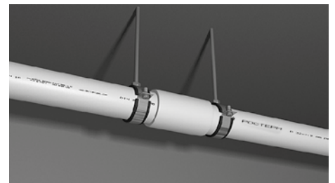
6. При помощи двух хомутов и одного фитинга
