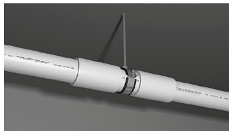
5. Между двумя фасонными изделиями
