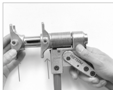
5. Переведите ручку тисков в верхнее положение, потяните вниз блокиратор, чтобы разъединить рычаг и насадку на тиски, вытащите осевые болты, установите необходимую насадку на тиски, зафиксируйте осевой болт и верните в исходное положение блокиратор
