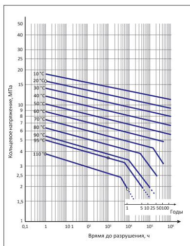
Рис. 1. Эталонные графики длительной прочности PP-R
