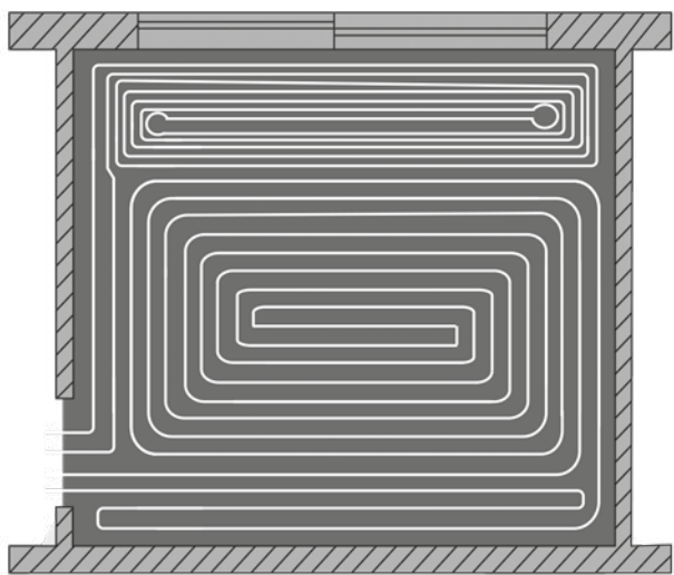
Укладка петель по принципу спирали
