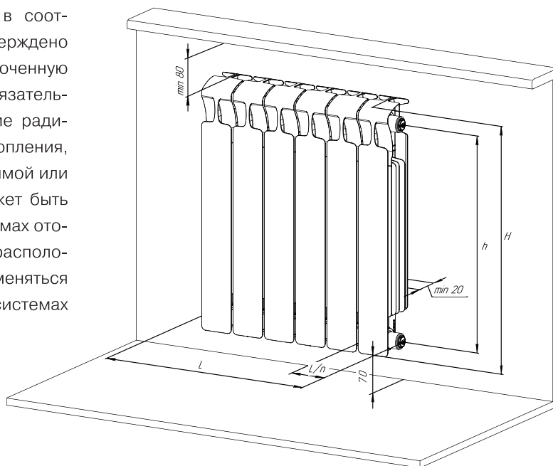
Рис 1. Схема настенного монтажа радиатора
