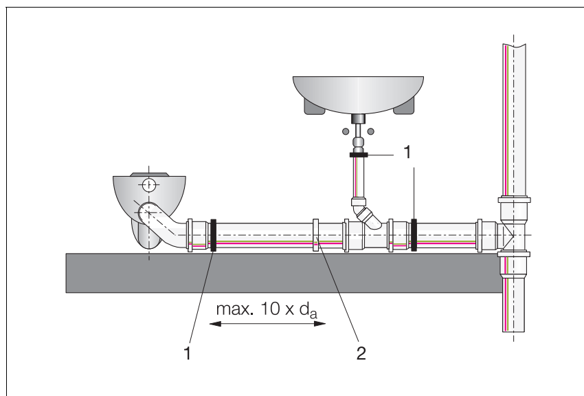
Рис. 4-6 Схема установки горизонтального трубопровода
