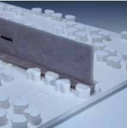
1 Рис. 43: Профиль деформационного шва и дополнительный профиль REHAU на матах с фиксаторами vario
