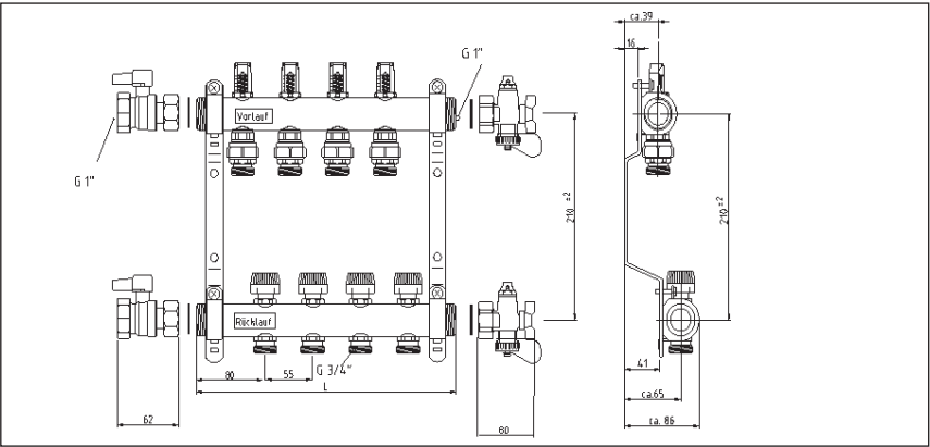
1 Рис. 55: : Присоединительные размеры распределительного коллектора НКV-D
