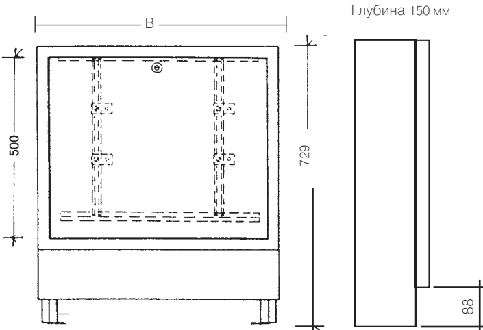
1 Рис. 58: Присоединительные размеры приставного распределительного шкафа
