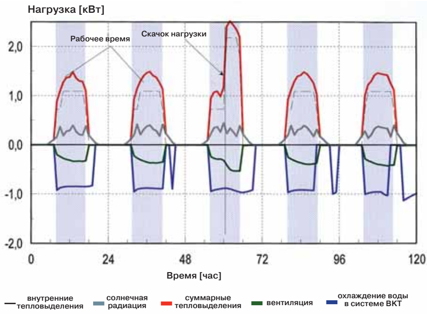
5 Рис. 39: График нагрузок в режиме охлаждения/Вариант А
