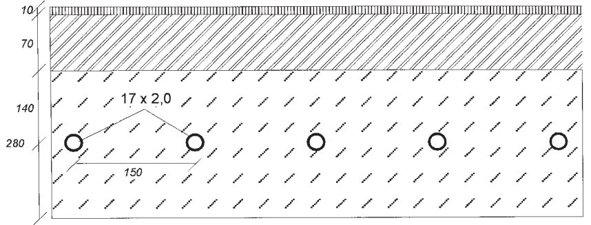
5 Рис. 43: Конструкция плиты перекрытия ВКТ в разрезе
