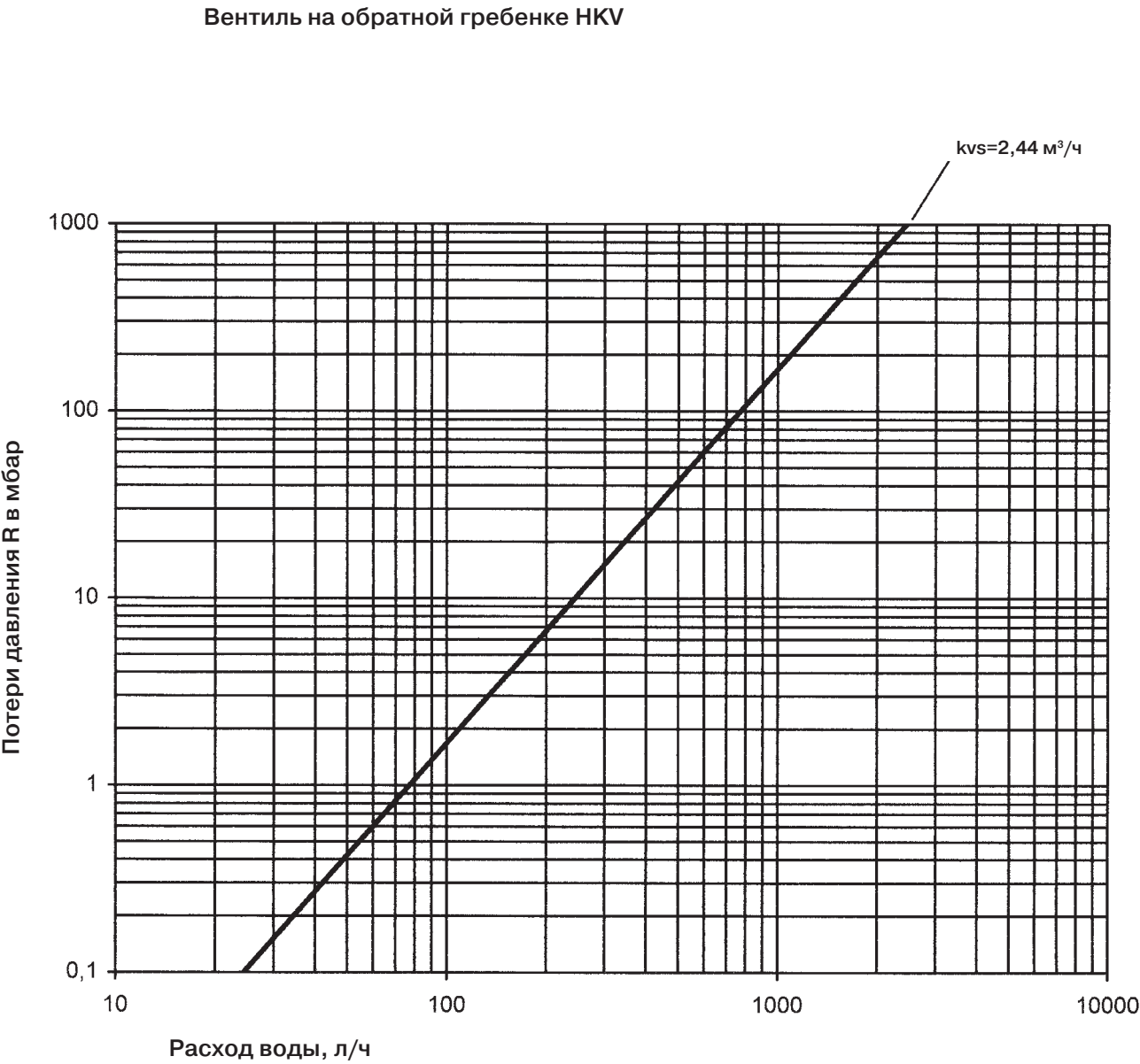
2 Рис. 4: Диаграмма расхода воды для вентилей на обратной гребенке -НКV
