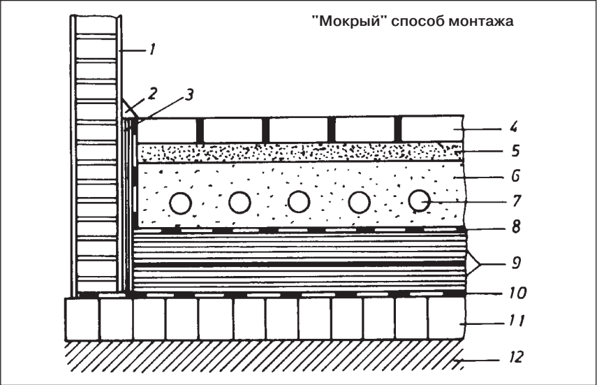
1 Рис. 76: Конструкция пола при "мокром" способе монтажа.
