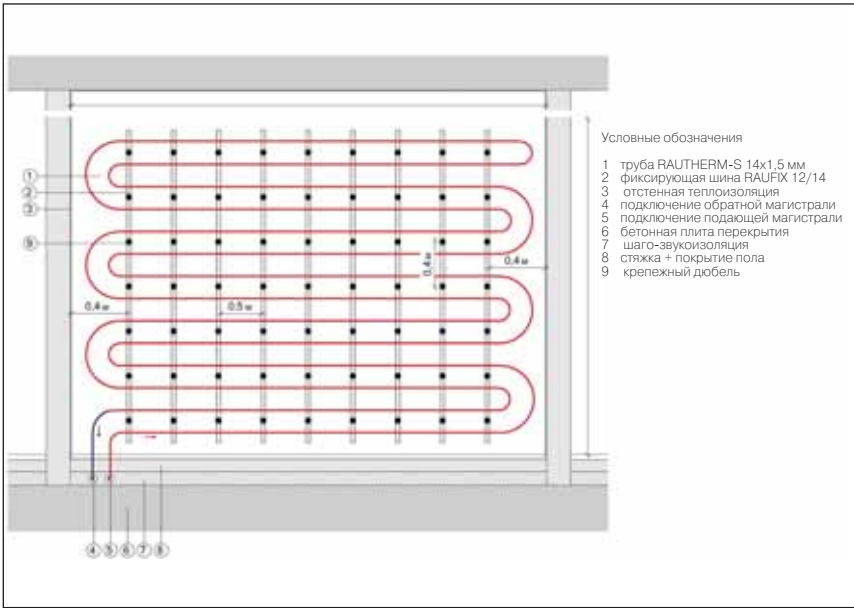
3 Рис. 16: Схематичное изображение системы настенного отопления REHAU с укладкой труб двойным змеевиком при "мокроем" способе монтажа
