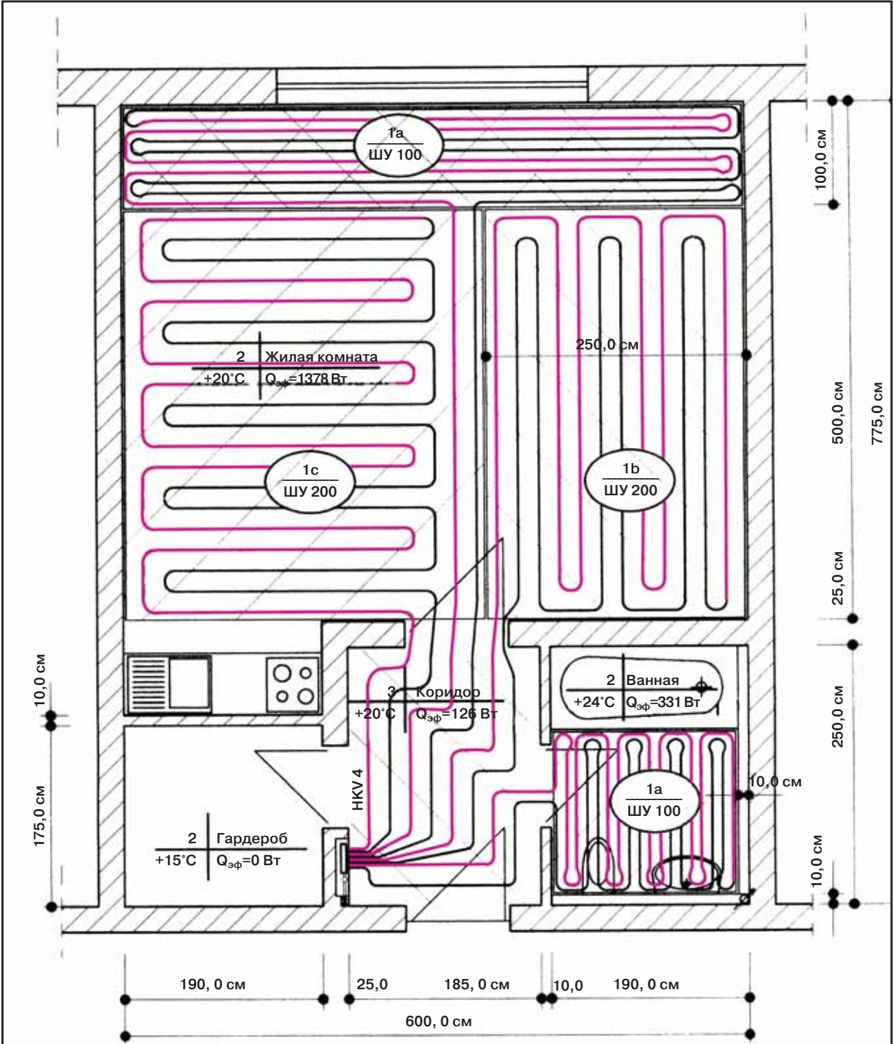
Пример расчета: План помещения с планом укладки труб
