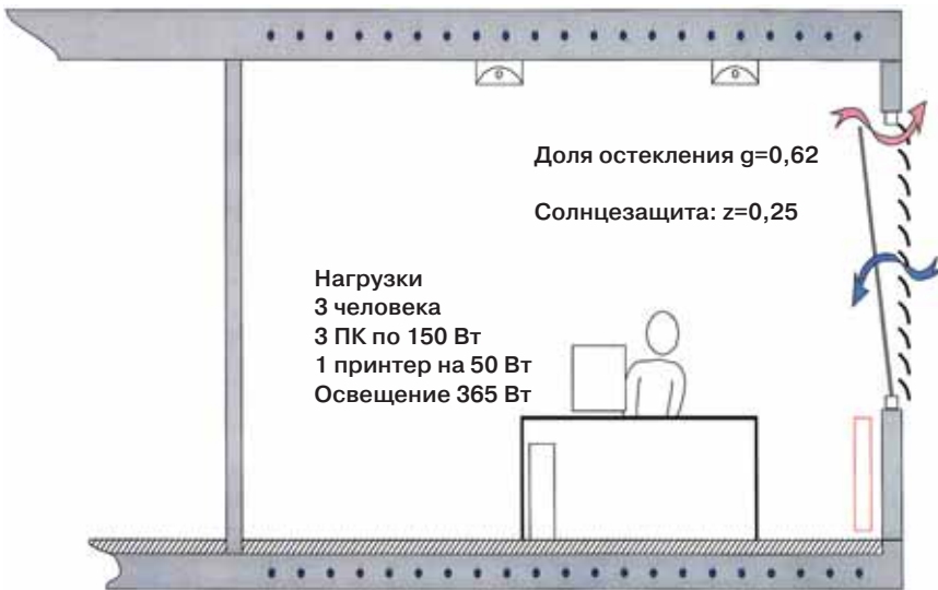
5 Рис. 42: Поперечный разрез по представительному помещению
