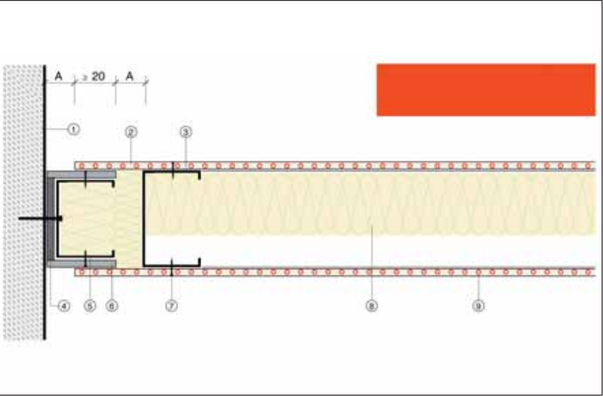
3 Рис. 35: Пример схемы скользящих швов примыкания фасадов
