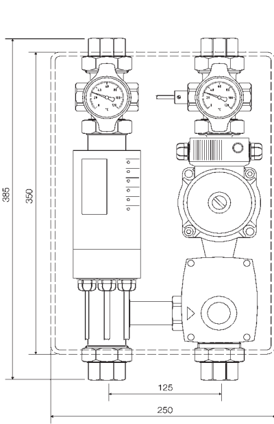
1 Рис. 65: Терморегулирующая станция TRS-20
