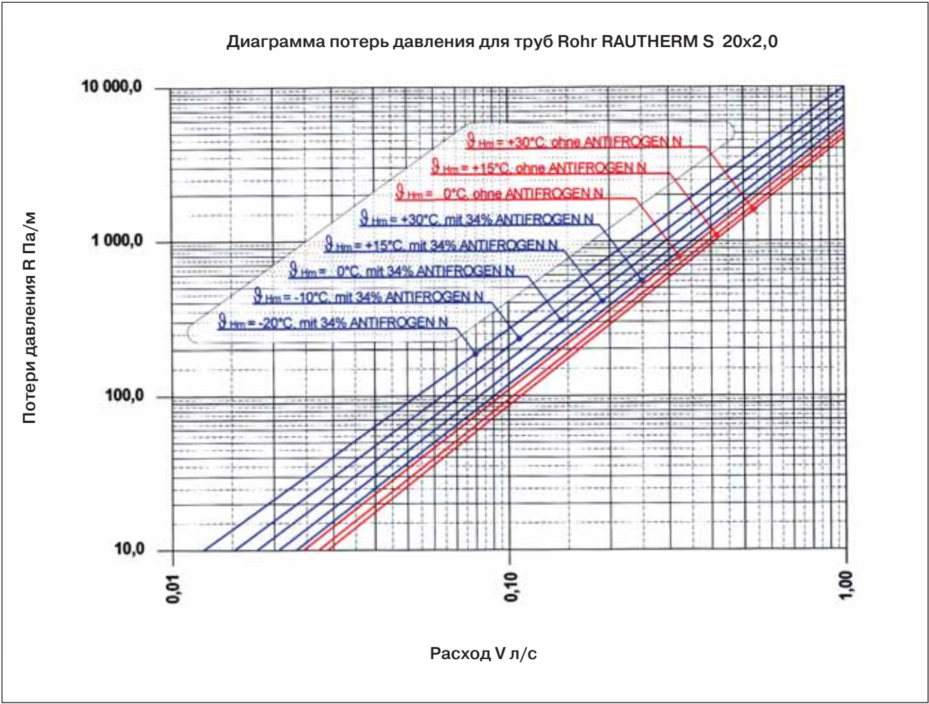
6 Рис. 30: Диаграмма потерь давления для систем с концентрацией антифригена 34%
