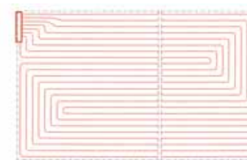
6 Рис. 12 Варианты укладки
