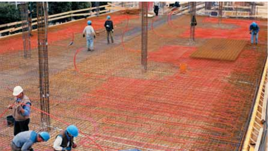
5 Рис. 5: Модули BKT REHAU, укладываемые на месте.
