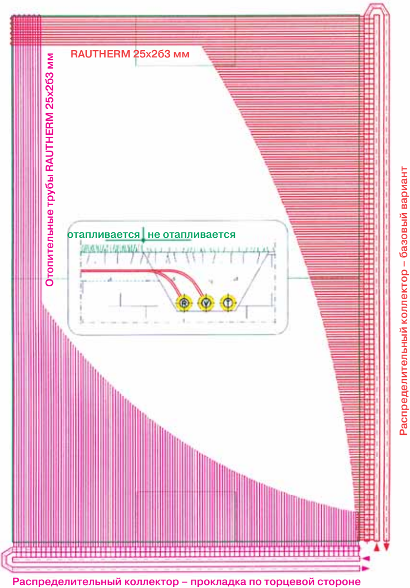
6 Рис. 31: Система обогрева футбольного поля RENAУ - схема укладки труб
