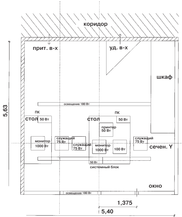
5 Рис. 34: План представительного помещения
