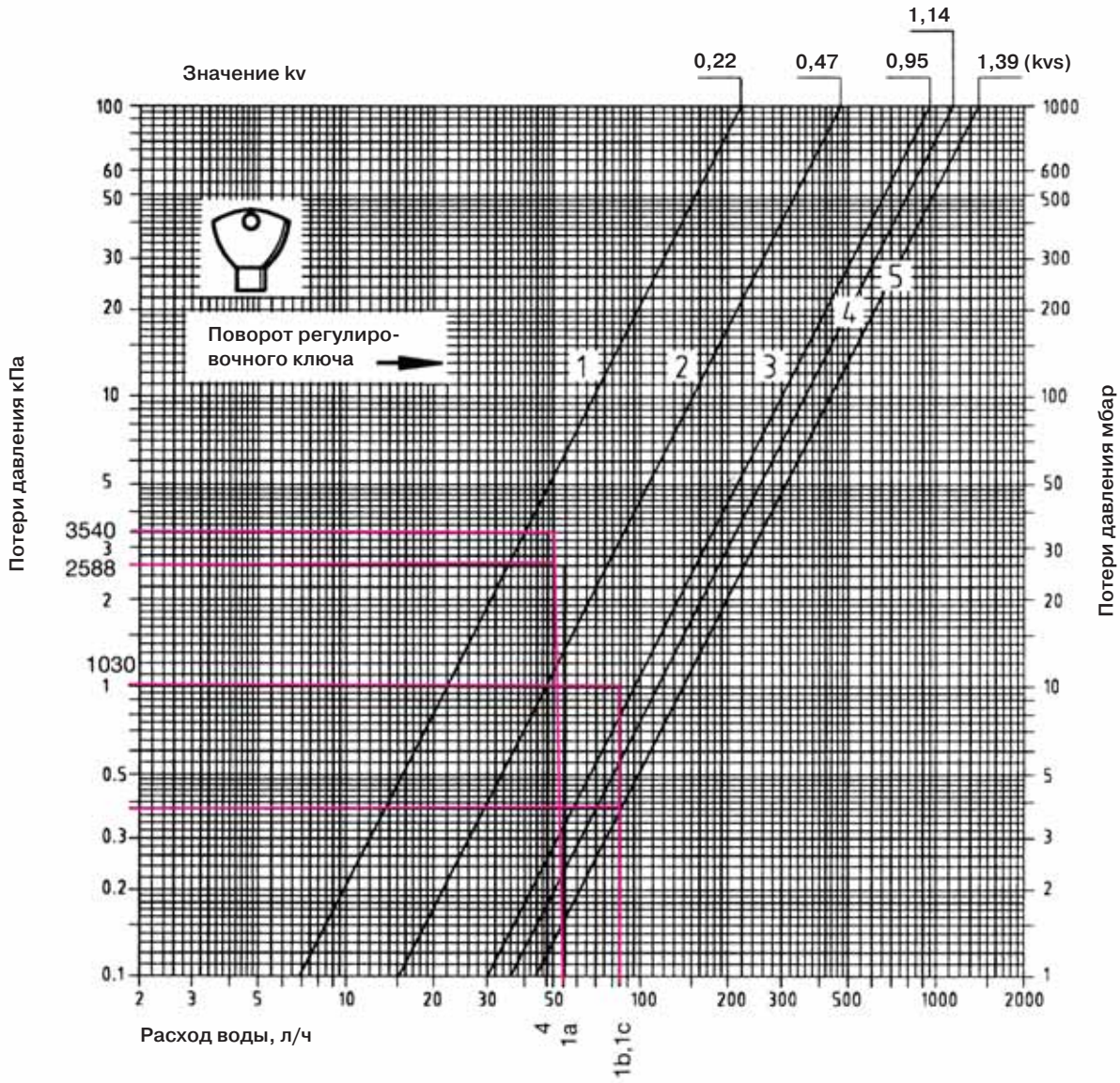
2 Рис. 4: Диаграмма расхода воды для вентилей тонкой регулировки - НКV
