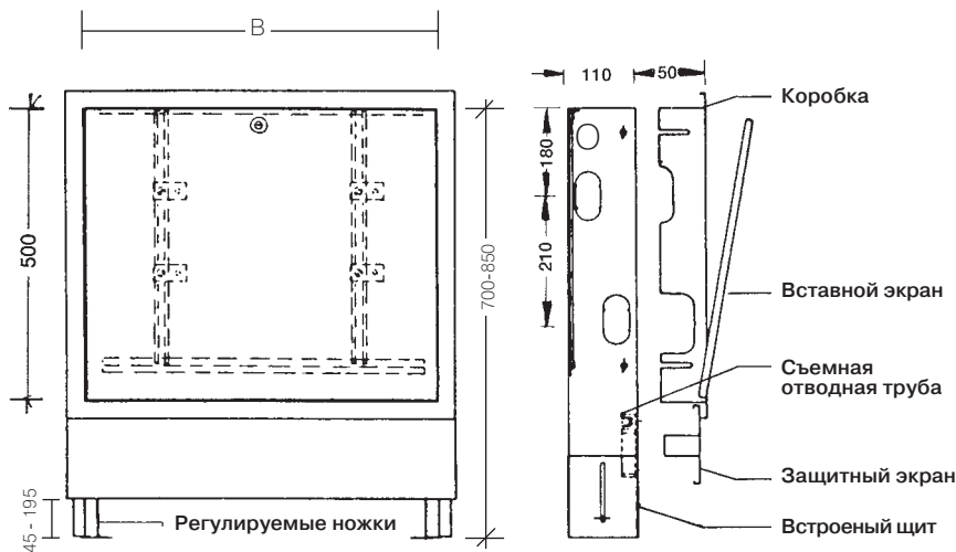
1 Рис 57: Присоединительные размеры встроенного распределительного шкафа
