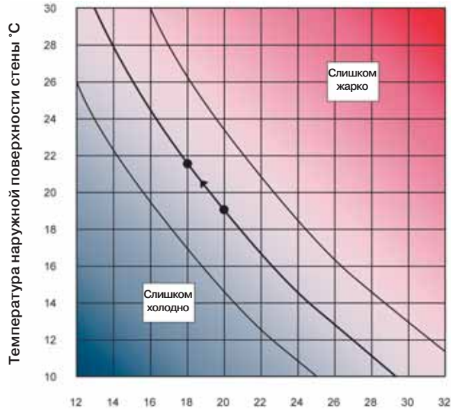
3 Рис. 2: Комфорт и низкая температура воздуха в помещении, система настенного отопления REHAU, экономящая энергию.
