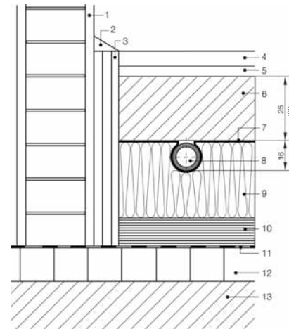
1. внутренняя штукатурка 2. плintус 3. оstenная теплоизоляция 4. плитка керамическая или из природного камня 5. мастика 6. сухая стяжка 7. теплопроводящая пластина, каширована на позиции 9 8. труба RAUTHERM S 9. монтажные плиты из вспененного полистирола PS 10. тепло- и звукоизоляция согласно DIN 4725, 4 109, WSchV 11. гидроизоляция (согласно DIN 18 195) 12. плита перекрытия 13. грунт
