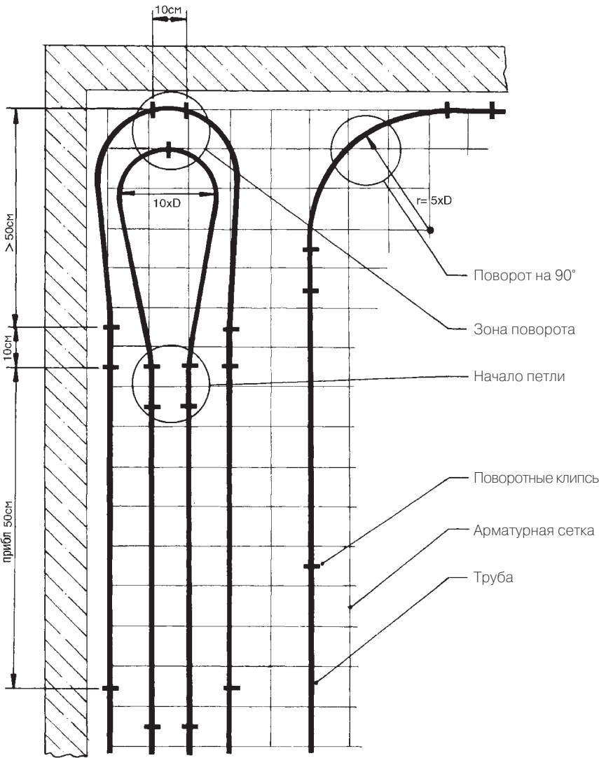
1 Рис. 33: Разворот и поворот труб в контуре
