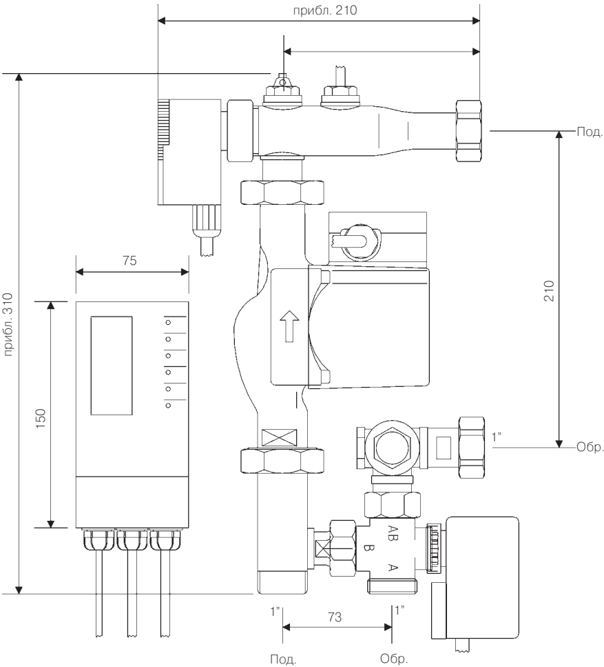
1 Рис. 71 : Размеры терморегулирующей станции TRS-T
