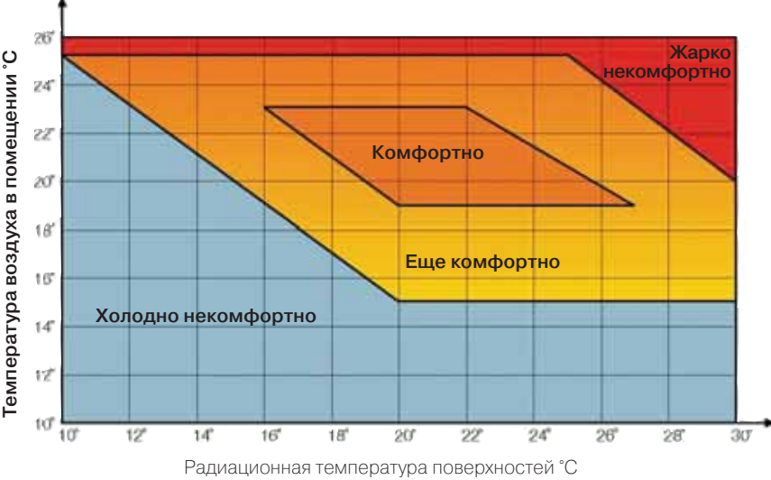
1 Рис. 7: Комфорт в зависимости от сочетания температур воздуха в помещении и радиационной температуры внутренних поверхностей
