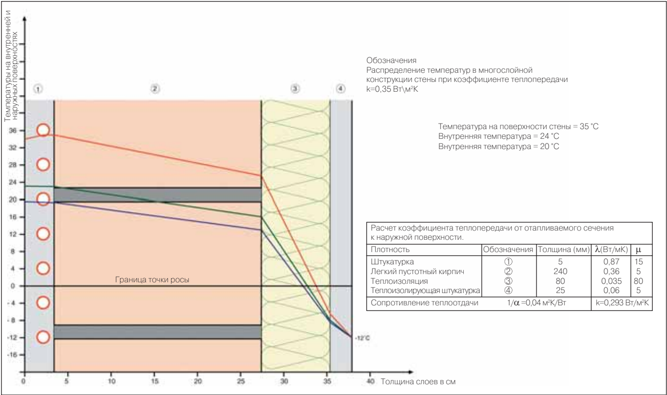
4 Рис. 1: Сравнение распределения температур в многослойной конструкции стены.
