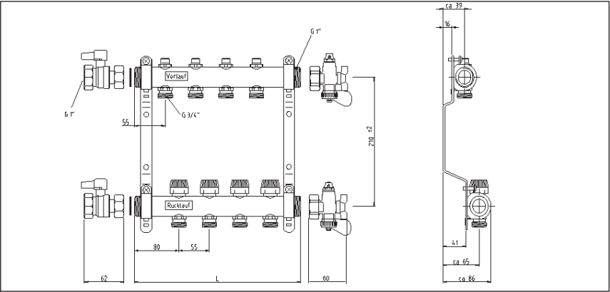
1 Рис. 54: Присоединительные размеры распределительного коллектора НКV
