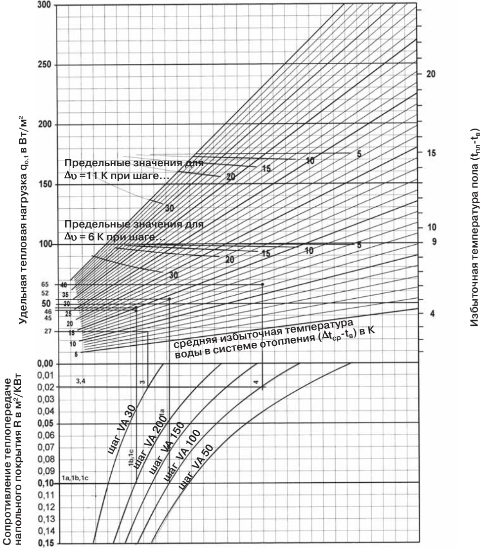
Диаграмма для определения нагрузки при укладке труб RAUTHERM S 17x2,0 мм RF, RAUTHERM S 17x2,0 мм
