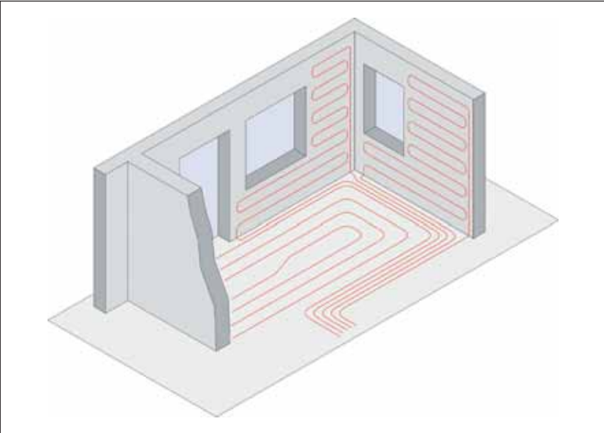
3 Рис. 8: Система настенного отопления REHAU в сочетании с системой напольного отопления/охлаждения
