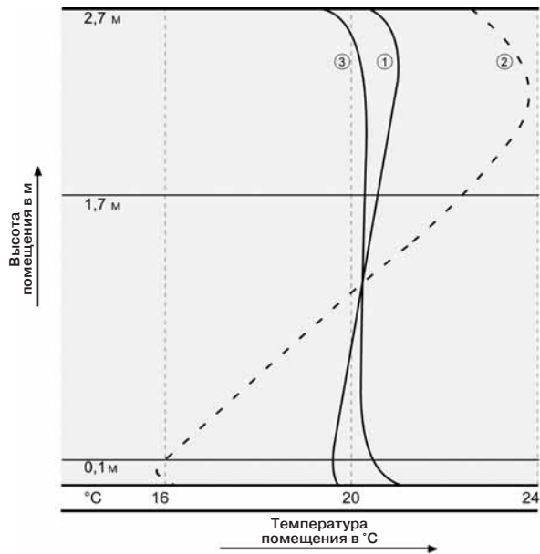
3 Рис. 3: Сравнение кривой распределения температур по высоте помещения при системе настенного отопления REHAU 1, традиционной системе отопления 2 с идеальной кривой распределения температур по высоте помещения 3
