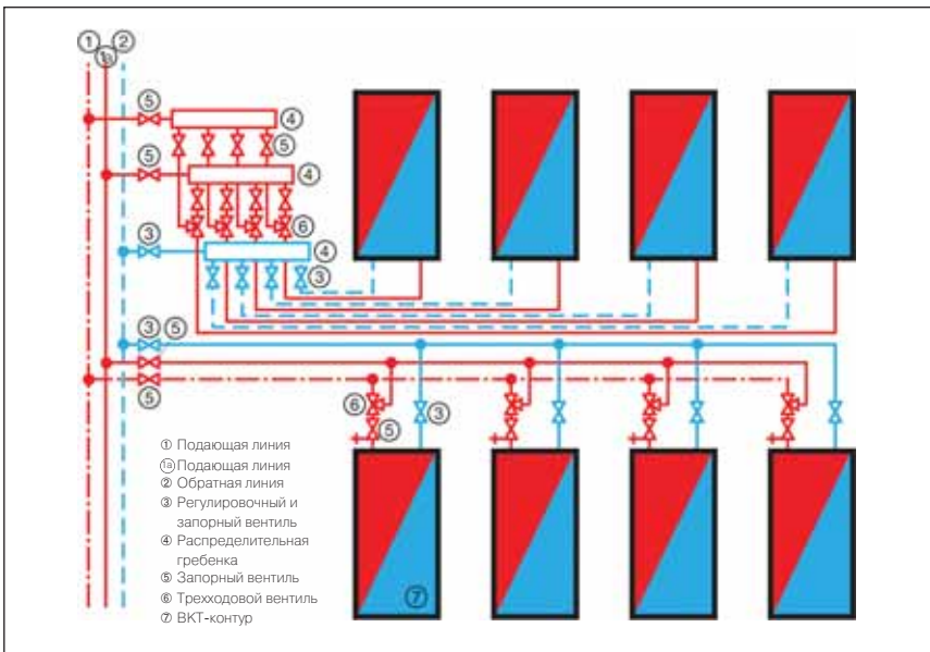
5 Рис. 52: Схематичное представление трехтрубной системы
