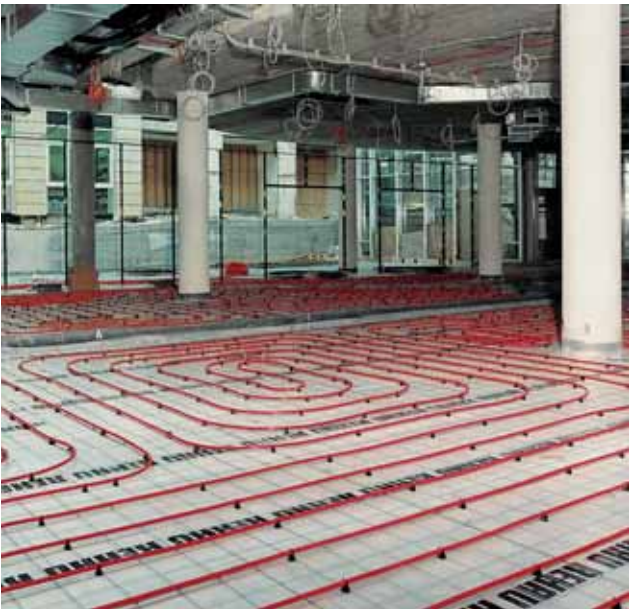
1 Рис. 4: Система крепления труб на арматурной сетке REHAU
