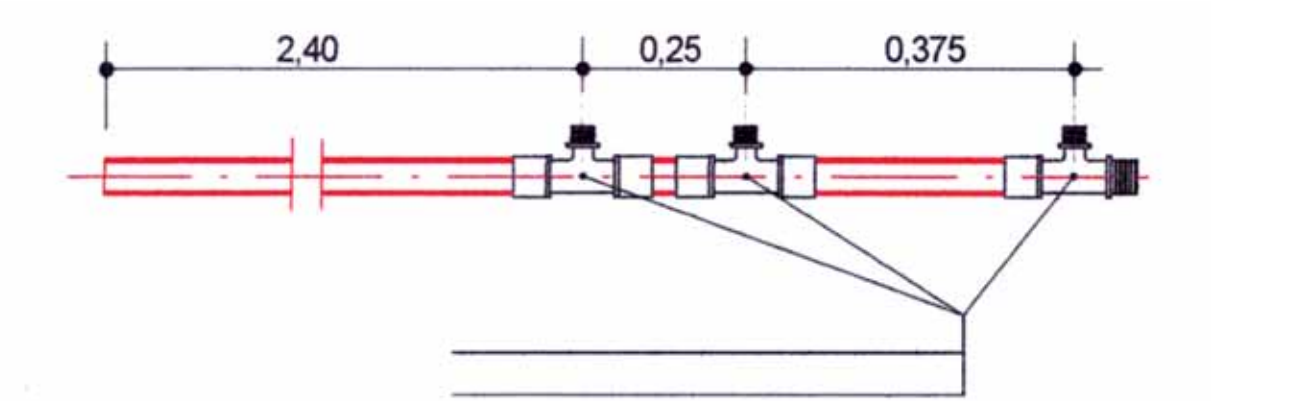
6 Рис. 23: Распределительный коллектор REHAU
