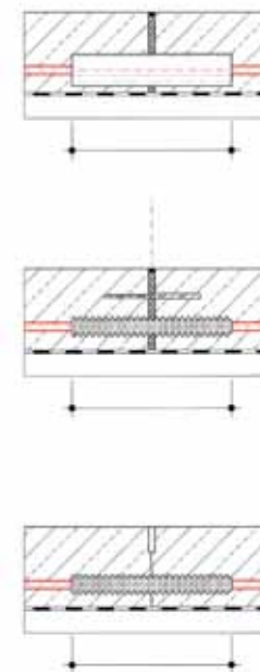
6 Рис. 11 Защита отопительных труб при пересечении ими температурного шва
