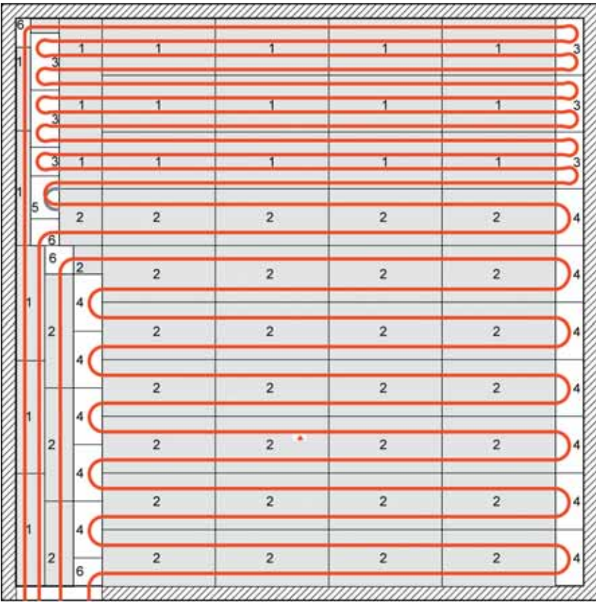
1 Рис. 39: Пример плана укладки плит при "сухом" способе монтажа REHAU
