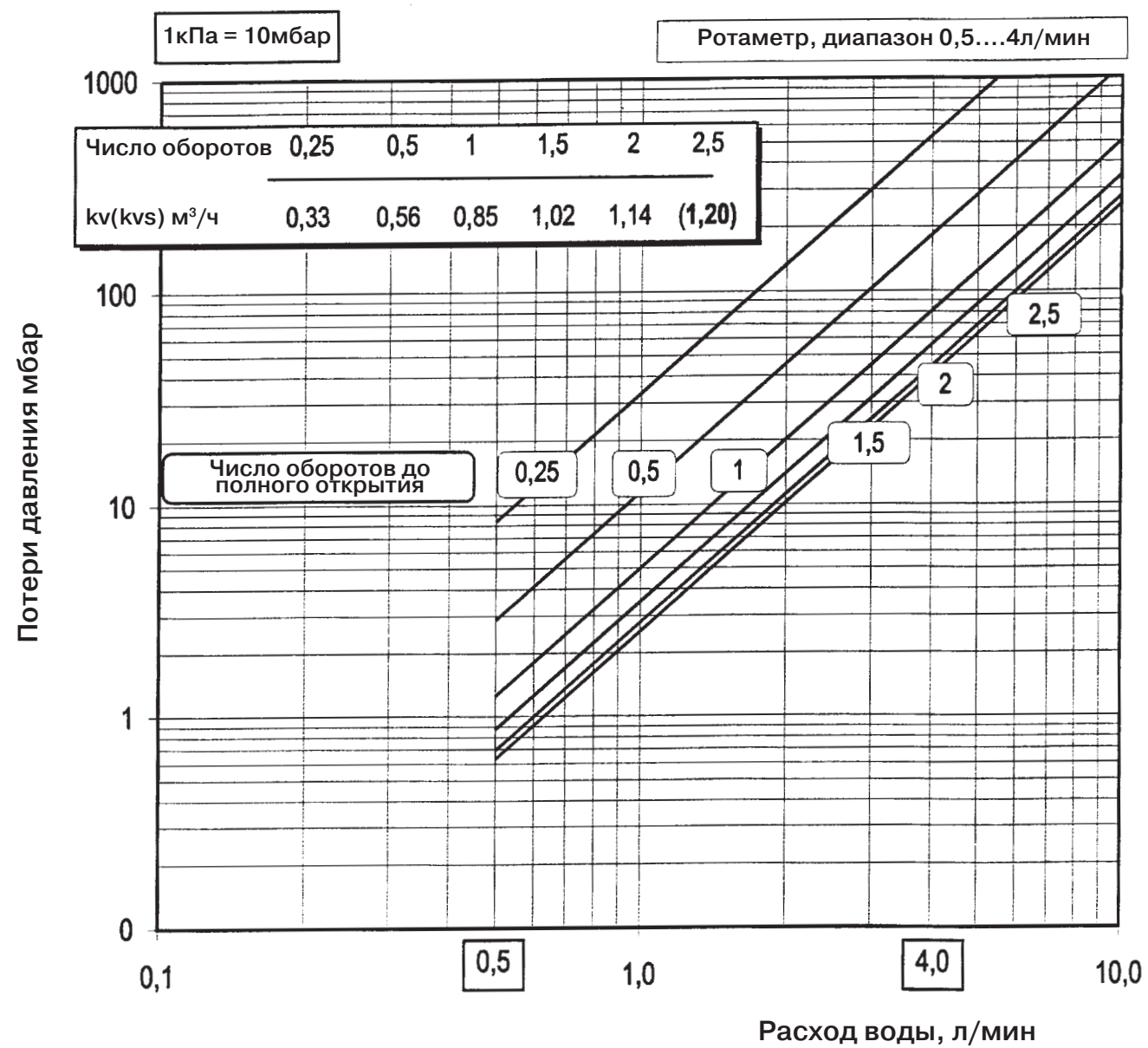
2 Рис. 6: Характеристики вентилей тонкой регулировки на распределительном коллекторе НКV-D
