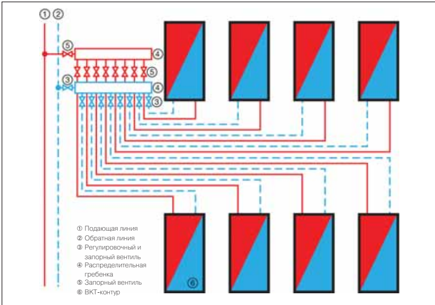
5 Рис. 50: Схема подключения к коллектору
