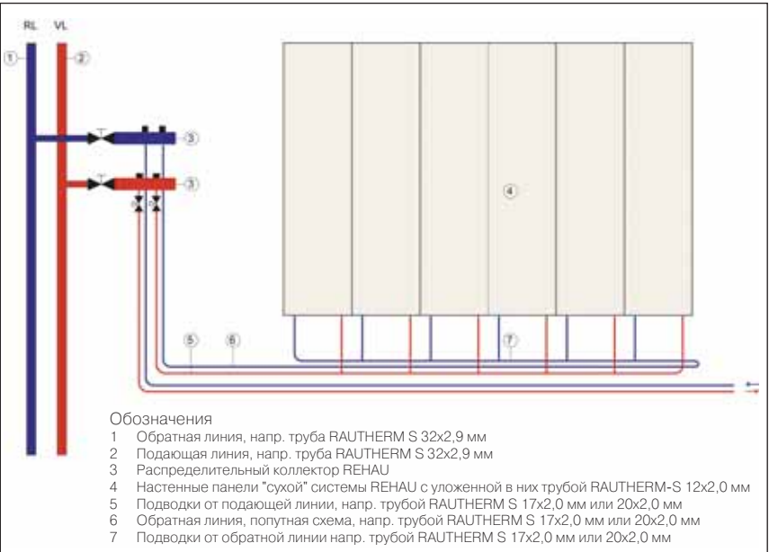
4 Рис. 4: Схематичное представление присоединения нескольких зон по попутной схеме
