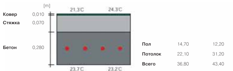
5 Рис. 48: Конструкция плиты 3
