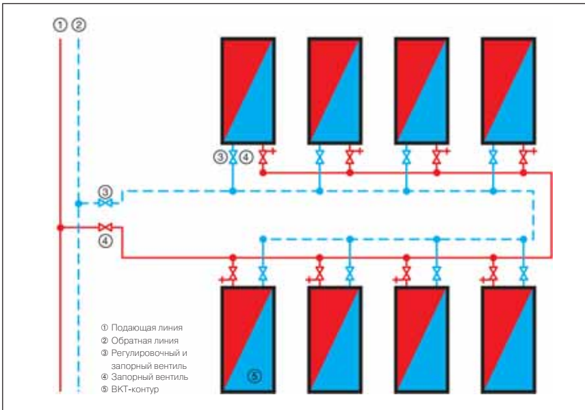
5 Рис. 51: Схематичное представление двухтрубной системы
