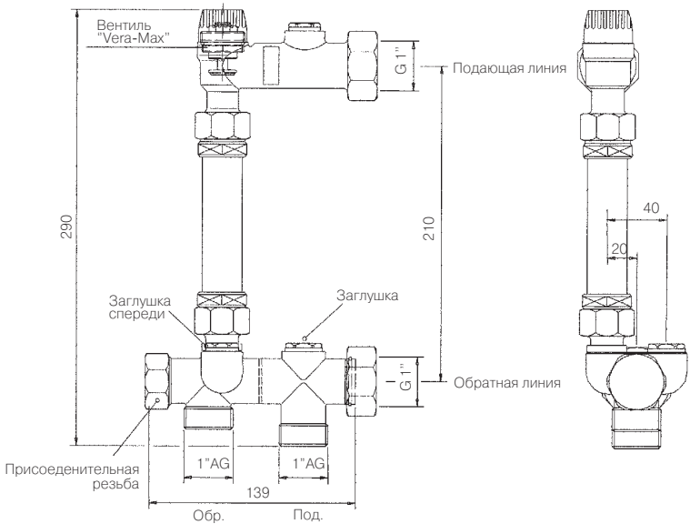
1 Рис. 61: Размеры комплекта для установки теплосчетчика REHAU
