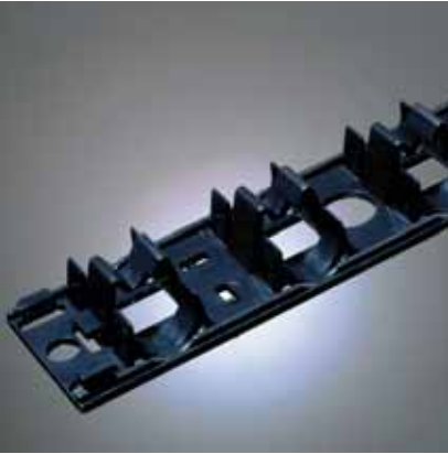
5 Рис. 16: Фиксирующая шина REHAU RAUFIX
