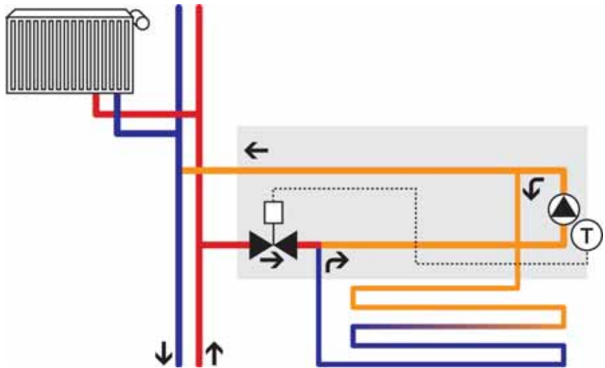
1 Рис. 69: Схема подключения
