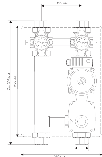
1 Рис.67: Смесительный узел PMG-25
