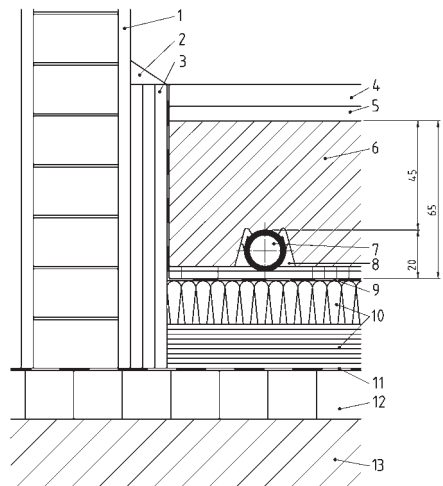
1. внутренняя штукатурка 2. плинтус 3. отстенная теплоизоляция 4. плитка керамическая или из природного камня 5. мастика 6. цементная стяжка согласно DIN 18560 7. труба RAUTHERM S 8. фиксирующая шина RAUFIX REHAU из PP 9. защитная пленка согласно DIN 18560, полиэтиленовая 10. пленка или пропитанная битумом бумага 11. тепло- и звукоизоляция согласно DIN 4725, 4109, WSchV 12. гидроизоляция (согласно DIN 18195) 13. плита перекрытия 14. грунт
