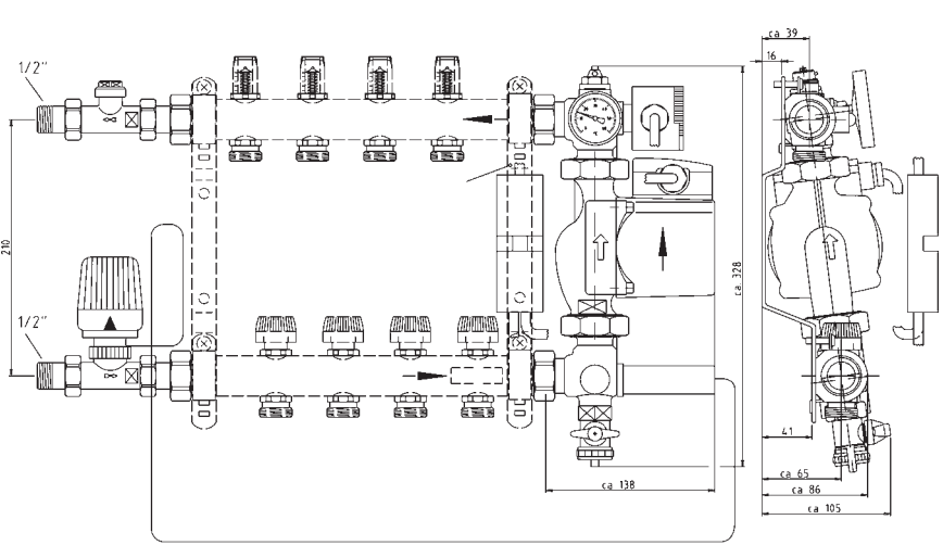
1 Рис. 68: Комплект температурного регулирования с постоянными параметрами
