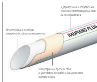
Рис. 18-1 Конструкция трубы RAUPIANO PLUS
