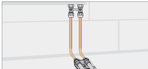
Рис. 14.3-3 Комплект Г-образных присоединительных трубок из меди
