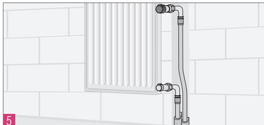
Рис. 14.4-10 Подключение к запорно-регулирующей арматуре радиатора при помощи Г-образных присоединительных трубок
