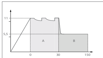
Рис. 17.2-8 Диаграмма гидравлического испытания для труб RAUTITAN flex, RAUTITAN his A Предварительное испытание (с доведением давления до испытательного) B Основное испытание систем из труб RAUTITAN flex, RAUTITAN his в возможной комбинации с трубами RAUTITAN stabil / RAUTITAN stabil platinum и со стальными трубами
