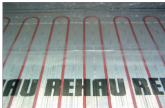
Рис. 15.6-1 Система укладки труб на теплоизоляционных матах TS-14
