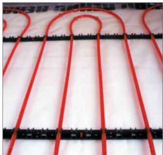
Рис. 15.5-7 Система RAUFIX
