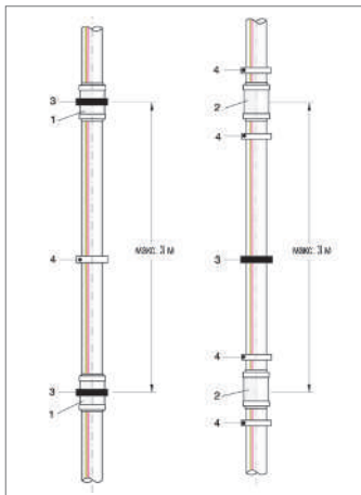
Рис. 18.1-2 Применение двухраструбных или надвижных муфт 1 Двухраструбная муфта 2 Надвижная муфта 3 Неподвижный хомут 4 Направляющий хомут
