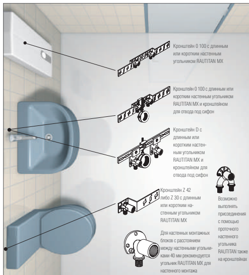
Рис.17.2-6 Кронштейны для гостевого санузла
