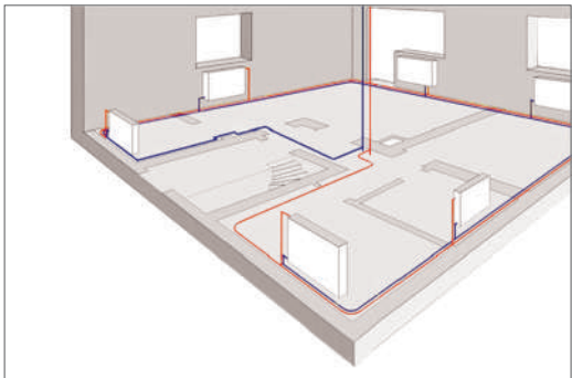
Рис. 14.1-3 2-х трубная горизонтальная попутная
