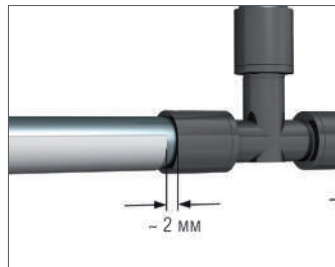
Рис. 9-5 Фиксирующий желоб недопустимо прокладывать поверх подвижных гильз RAUTITAN PX
