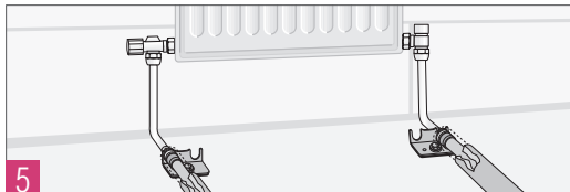
14.3-10 Подключение отопительного прибора при помощи Г-образных присоединительных трубок
