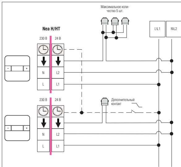
Рис. 15.8-7. Схема электрического подключения терморегуляторов NEA H и NEA HT без применения клеммной колодки
