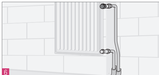
Рис. 14.4-12 Подключение к запорно-регулирующей арматуре радиатора с помощью переходника с наружной резьбой RAUTITAN RX
