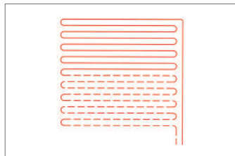
Рис. 15.4-2 Укладка змеевиком
