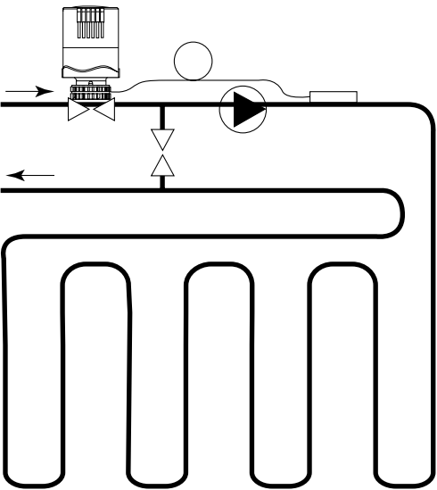
Теплый пол
