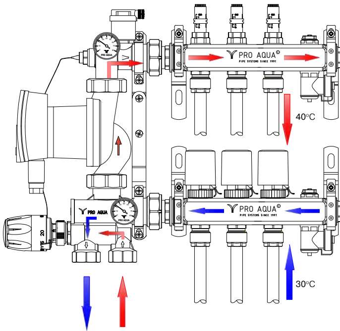
Схема движения теплоносителя
