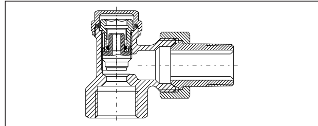
Разрез „Combi 3“ углового, с внутрен. резьбой по EN 10226-1
