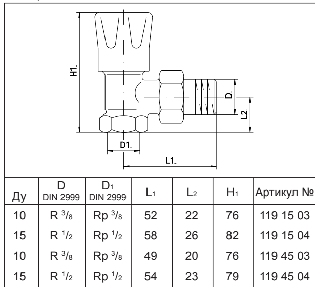
Угловой вентиль
