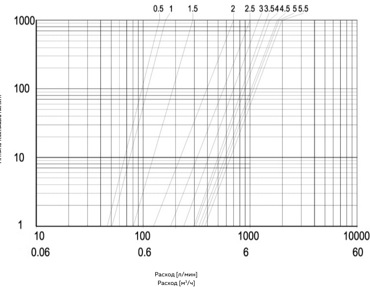
Диаграмма потерь давления
