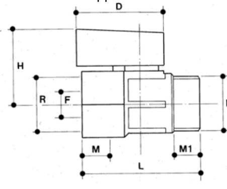
Соединение НВ
