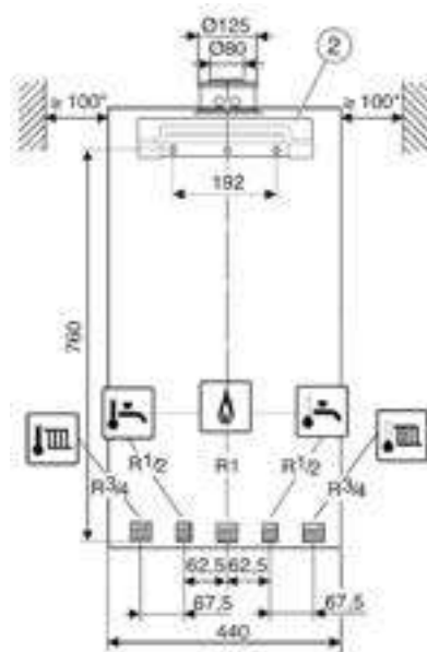
Размеры для GB172i-20..24
