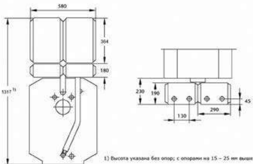
KAS 1/G125 c HKV 2/25
