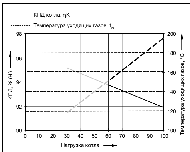
Схема 06: КПД котла и температура уходящих газов с учетом нагрузки котла при средней температуре воды в котле, равной 70^{\circ}\text{C}
