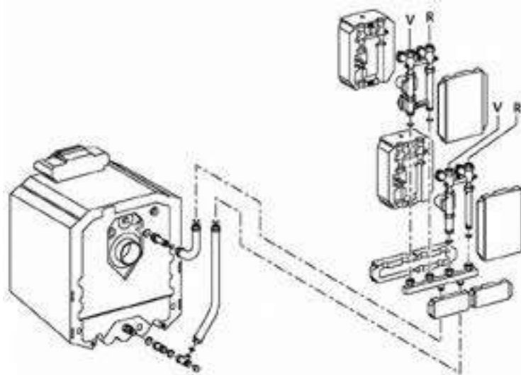
KAS 1/G125 c HKV 2/25
