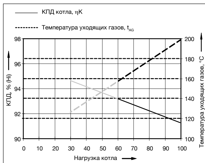
Схема 03: КПД котла и температура уходящих газов с учетом нагрузки котла и средней температуры воды в котле, равной 70^{\circ}\text{C}
