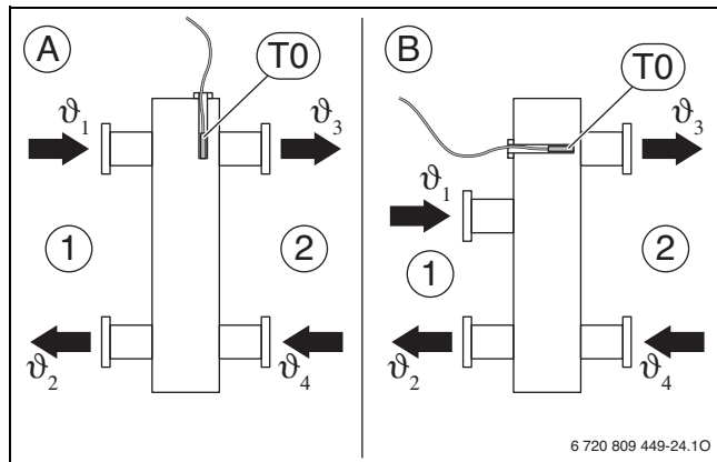
Sl. 4 Položaj tipala temperature dvižnega voda (T0)
