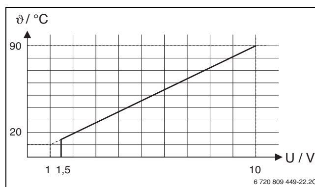
sl. 2 Linearna zavisnost između signala od 0-10 V (napon u voltima) i potrebne temperature polaznog voda \theta (u °C u odnosu na opseg od minimalne temperature polaznog voda do maksimalne temperature polaznog voda [osnovno podešavanje 20 °C do 90 °C])
