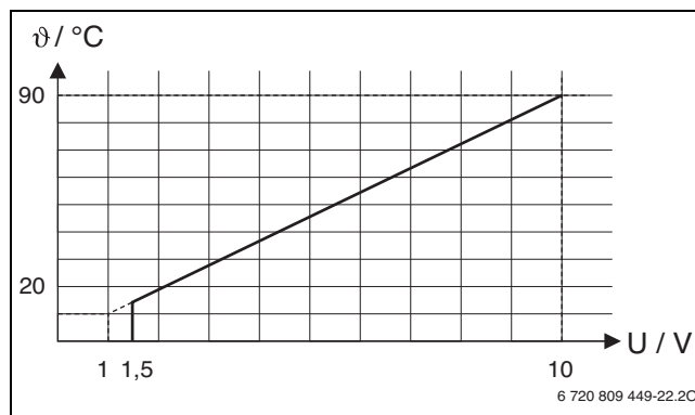
2. ábra Lineáris összefüggés a 0-10 V-os jel ( U fesz. V-ban) és az igényelt előremenő hőmérséklet között ( \theta °C-ban a minimális előremenő hőmérséklettől a maximális előremenő hőmérsékletig tartományra vonatkoztatva [alapbeállítás 20 °C ... 90 °C])
