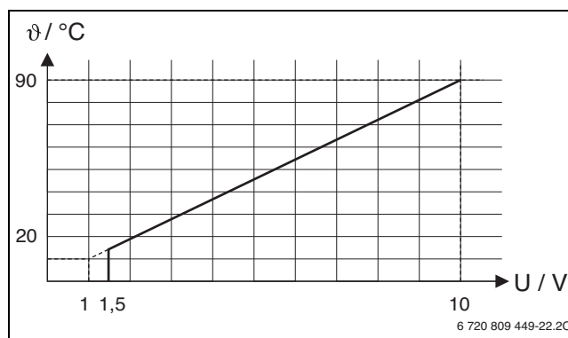
Sl.2 Linearna zveza med signalom 0–10 V ( U v Voltih) in zahtevano temperaturo dviznega voda \theta (v °C glede na območje od minimalne do maksimalne temperature dviznega voda [osnovna nastavitvev 20 °C do 90 °C])
