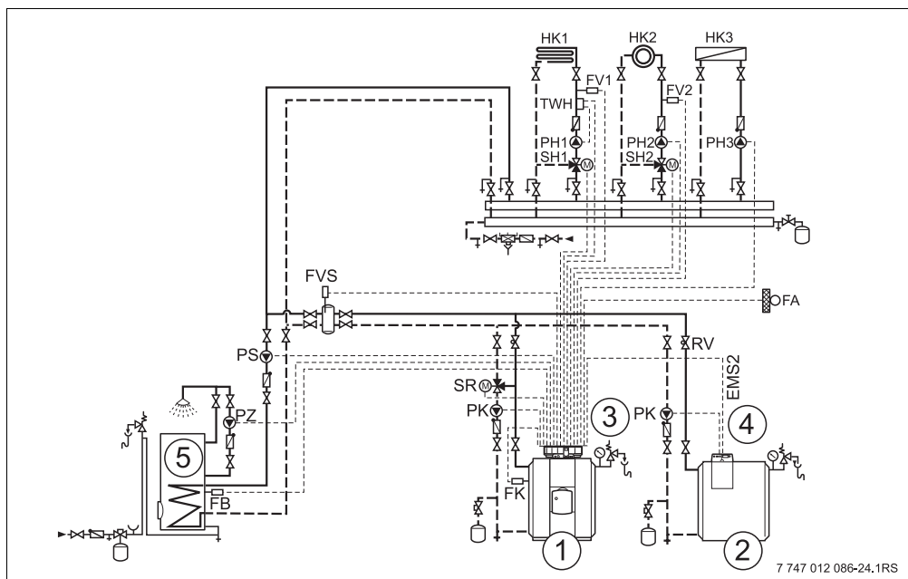
Рис. 21 Гидравлическая схема 8
