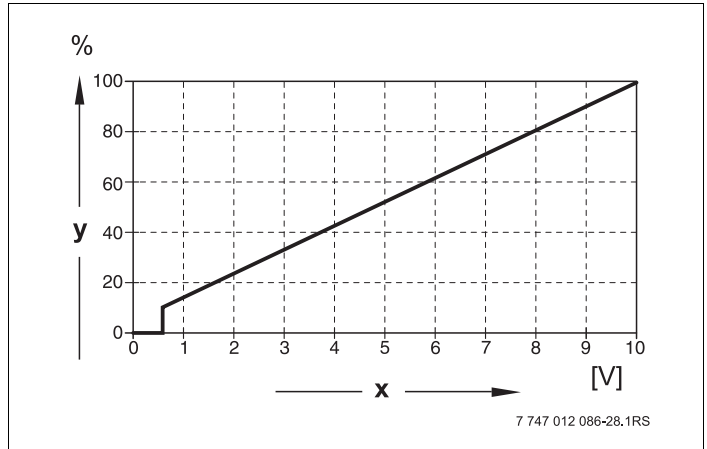
Рис. 26 Вход 0 – 10 В
