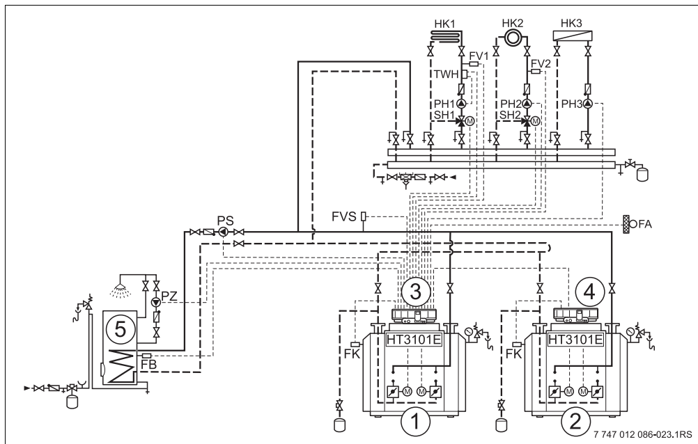
Рис. 20 Гидравлическая схема 7
