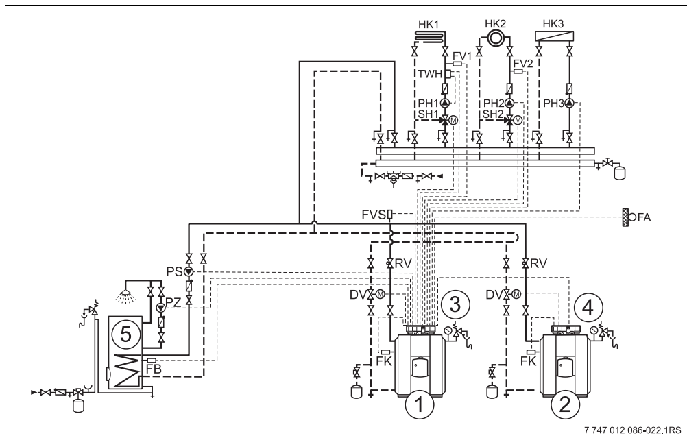
Рис. 19 Гидравлическая схема 6
