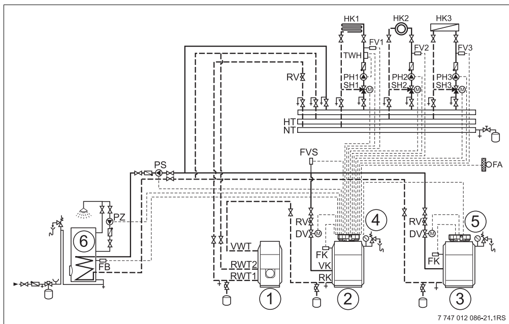
Рис. 18 Гидравлическая схема 5
