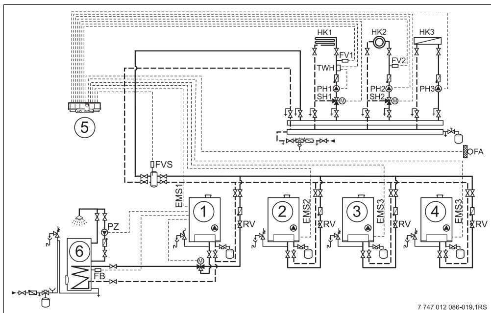
Рис. 16 Гидравлическая схема 3
