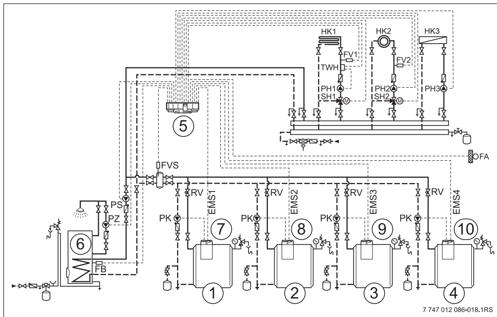
Рис. 15 Гидравлическая схема 2
