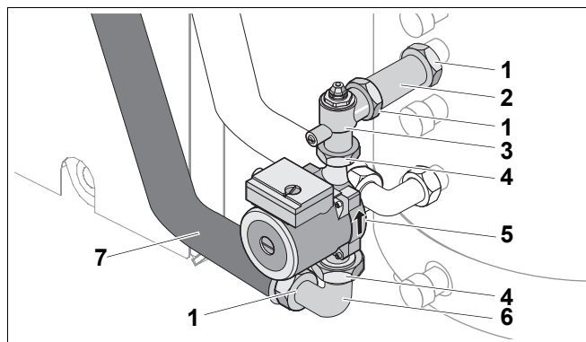
Рис. 8 Монтаж трубопровода на баке-водонагревателе
