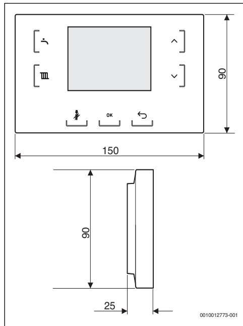
Рис. 1 Размеры, мм
