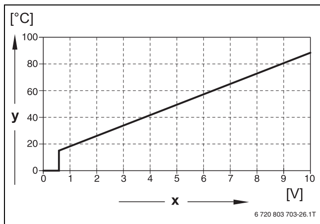
Рис. 22 У-клеммы 3 и 4
